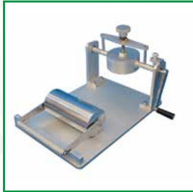
Dụng cụ test Cobb Cobb test instrument
